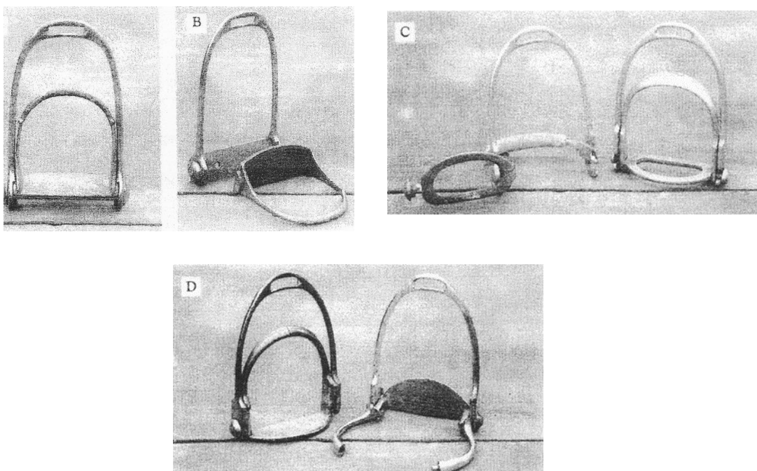
Rys. Rodzaje bezpiecznych strzemion
